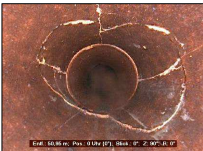
Abb.: Kanalkamerabild einer defekten Leitung (Scherbenbildung)
