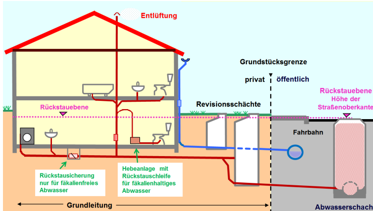
Abb.: die „Rückstauhöhe“ ist im Regelfall die Straßenebene. Bei einer Überlastung oder im Havariefall kann das Abwasser im öffentl. Kanal bis zum Deckelrand ansteigen und somit in den Anschluss zurückstauen. Die Entlüftung der Abwasserrohre auf dem Dach wird oft mit einem kleinen Schornstein verwechselt.
